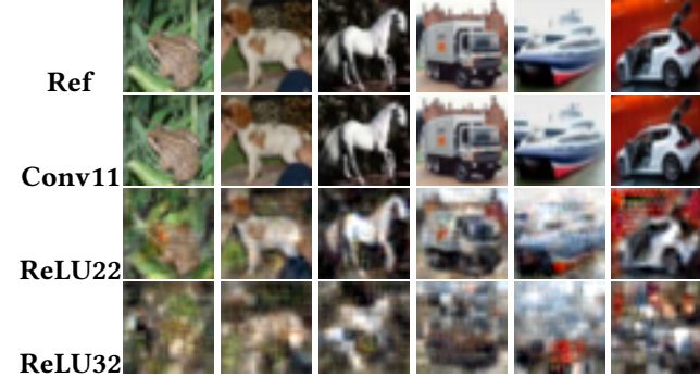
(b) CIFAR10.
