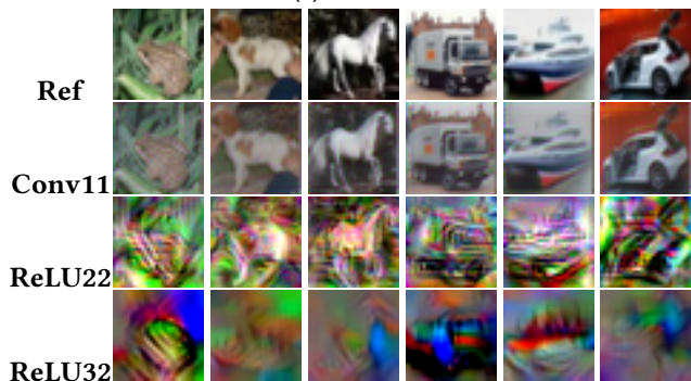
(b) CIFAR10.
