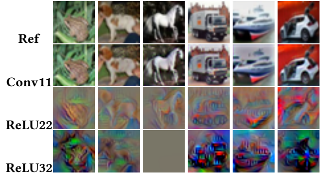
(b) CIFAR10.
