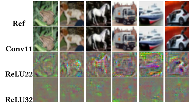
(b) CIFAR10.
